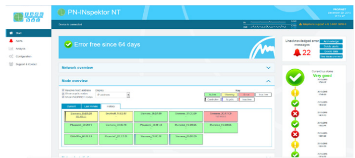
Web interface
